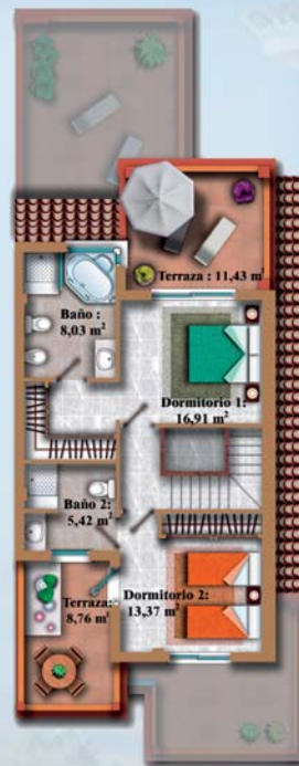
Planta Atico
